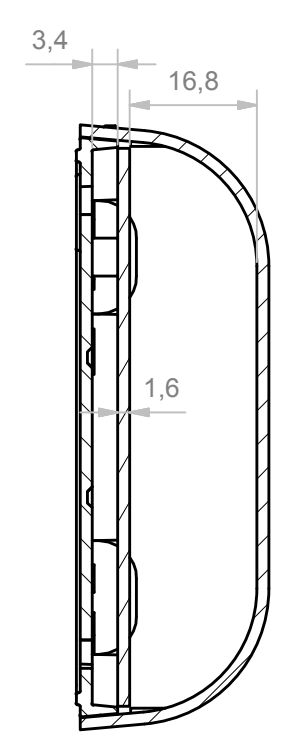
A-A (1:1)
